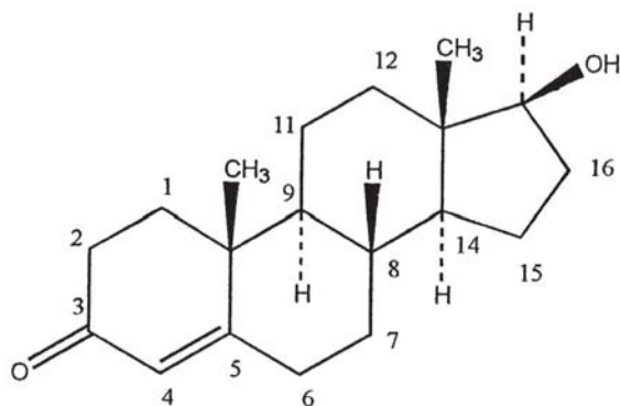
FIGURA 20.11-1 Estrutura molecular da testosterona.
